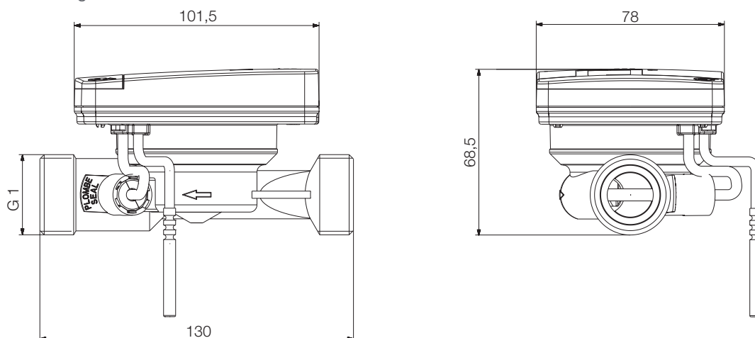
Einbaulänge 130 mm
