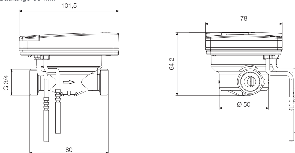
Einbaulänge 80 mm
