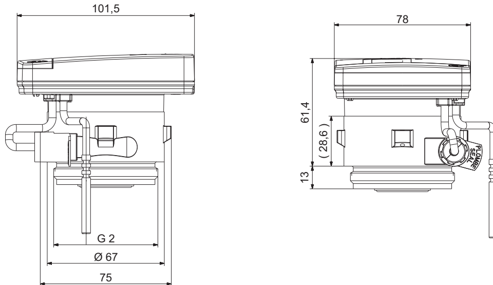
2"-Kapselzähler
