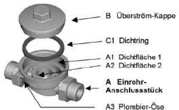
Abb. 1 Einrohranschlussstück
